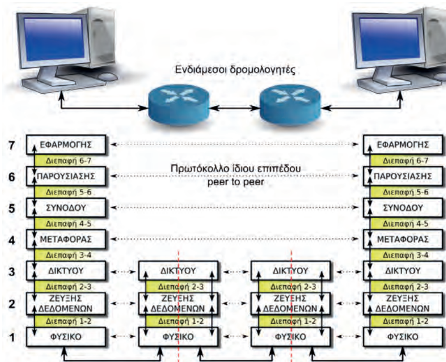
Εικόνα 1.2.1.β: Διαστρωματωμένη αρχιτεκτονική, διεπαφές και ομότιμα επίπεδα
