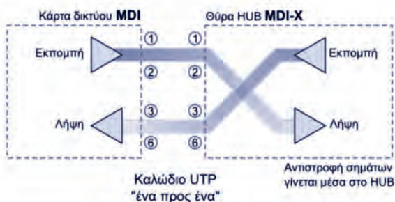
Εικόνα 2.4.3.α: MDI/MDI-X
