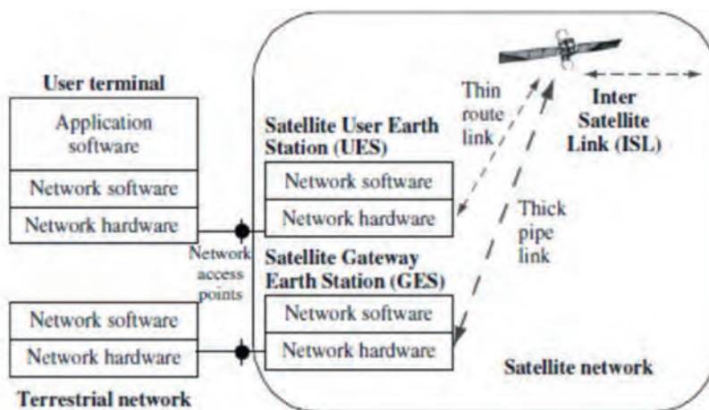
Σχήμα 5.3.2.β Σχέση επίγειου, δορυφορικού δικτύου και τερματικού χρήστη
