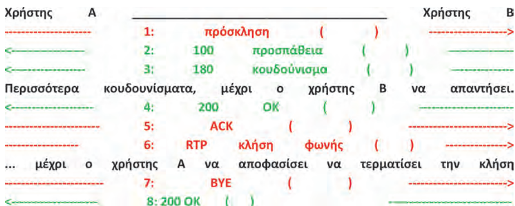
Σχήμα Π.5.α: Βήματα SIP κλήσης
