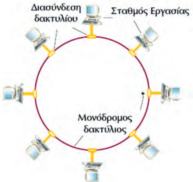
Σχήμα Π.1.δ. Δίκτυο δακτυλίου με κουπόνι
