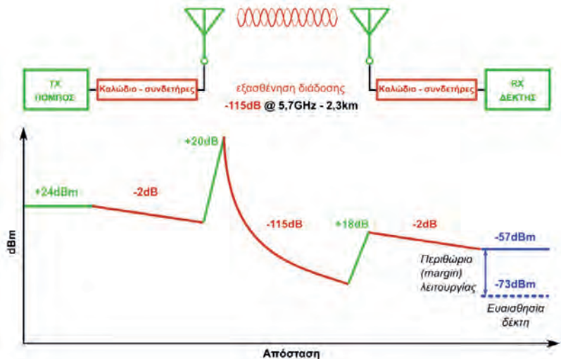
Εικόνα Π.2.α: Προϋπολογισμός ζεύξης (Link budget)
