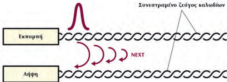
Εικόνα 2.4.1.ι: Παραδιαφωνία NEXT (Near End CrossTalk)
