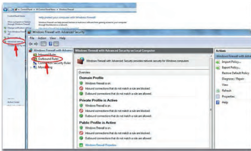
Εικόνα 5: Windows Firewall
