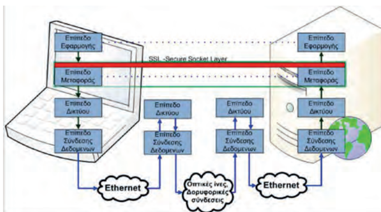
Εικόνα 8.2.3.β: Διαστρωμάτωση TCP/IP με TLS
