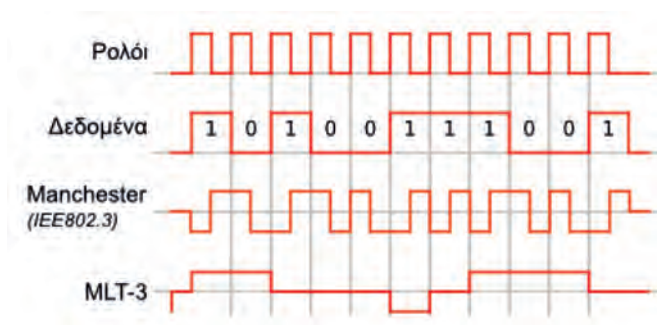
Εικόνα 2.4.1.κζ: Κωδικοποίηση Manchester, MLT-3
