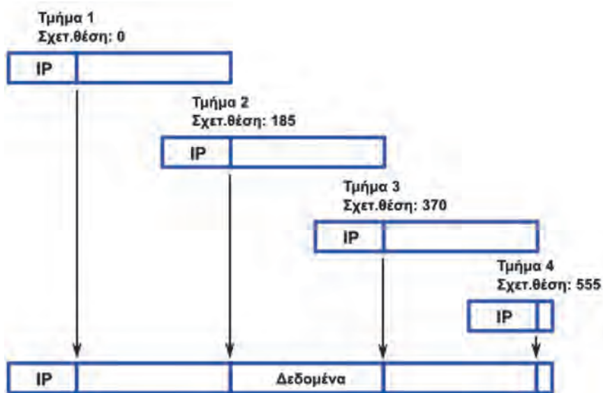
Εικόνα 3.2.δ: Επανασύνθεση κατατμημένου πακέτου IPv4
