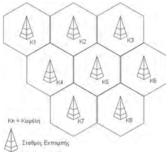
Σχήμα 2.5.α: Δίκτυο με κυψέλες
