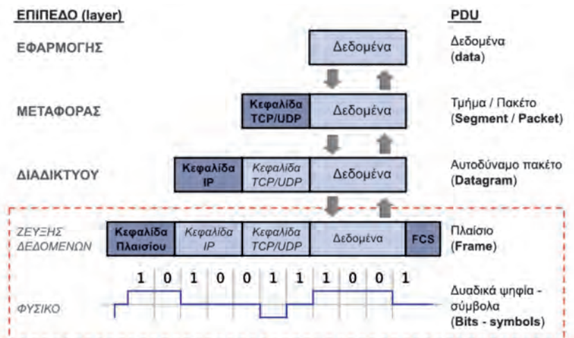
Εικόνα 1.3.α: Ενθυλάκωση
