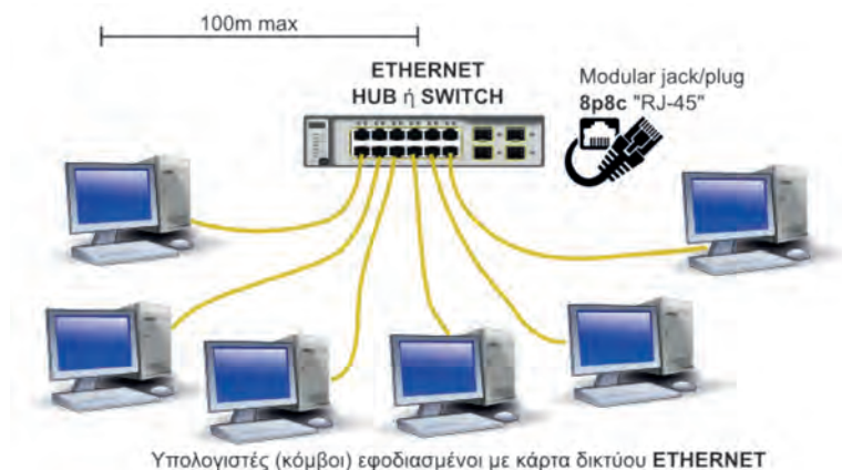
Εικόνα 2.4.1.στ: Δίκτυο Ethernet με χρήση καλωδίων συνεστραμμένων ζευγών.
