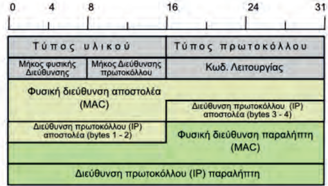
Εικόνα 3.3.β: Δομή πακέτου ARP
