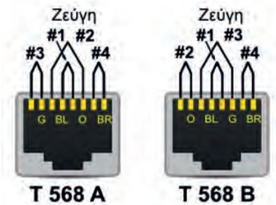
Εικόνα 2.4.1.κα: Συρμάτωση
