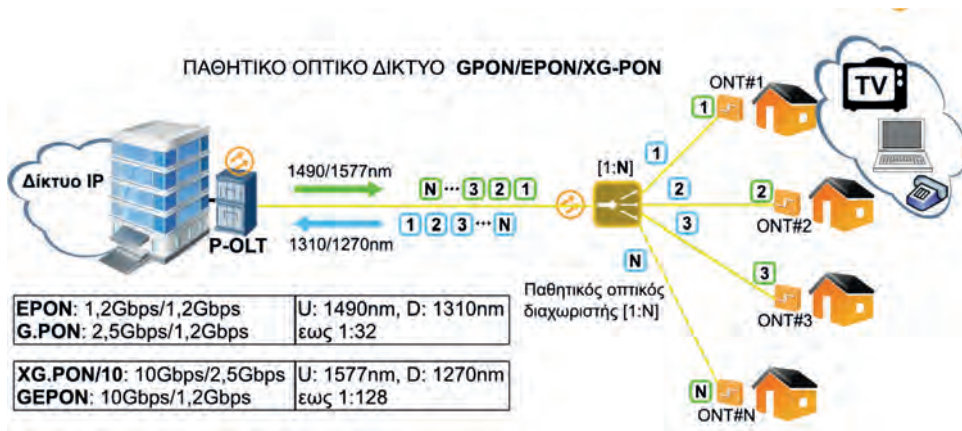
Εικόνα 5.2.ε: Παθητικό οπτικό δίκτυο (PON)
