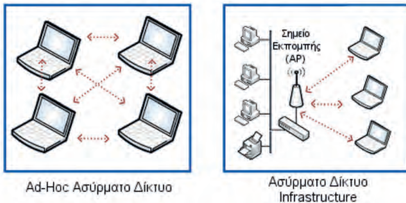
Εικόνα 2.5.2.α: Διαφορά ασύρματων τοπολογιών Ad-Hoc και Infrastructure
