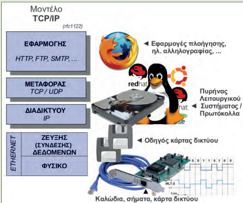
Εικόνα 1.2.2.β: Επίπεδα TCP/IP και αντίστοιχο Υλικό - Λογισμικό
