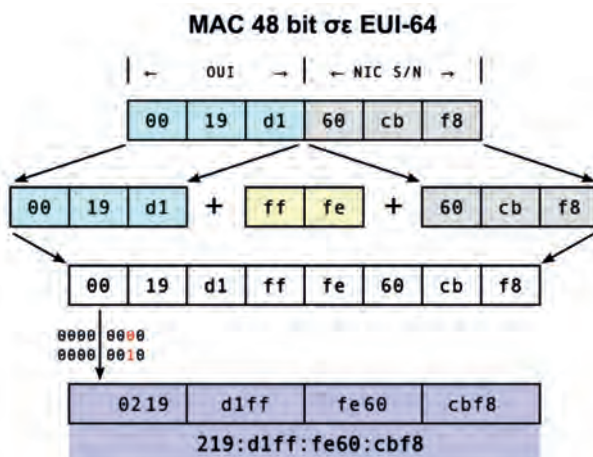
Εικόνα 3.5.1.α: Μεταγραφή διεύθυνσης MAC 48 bit σε EUI-64
