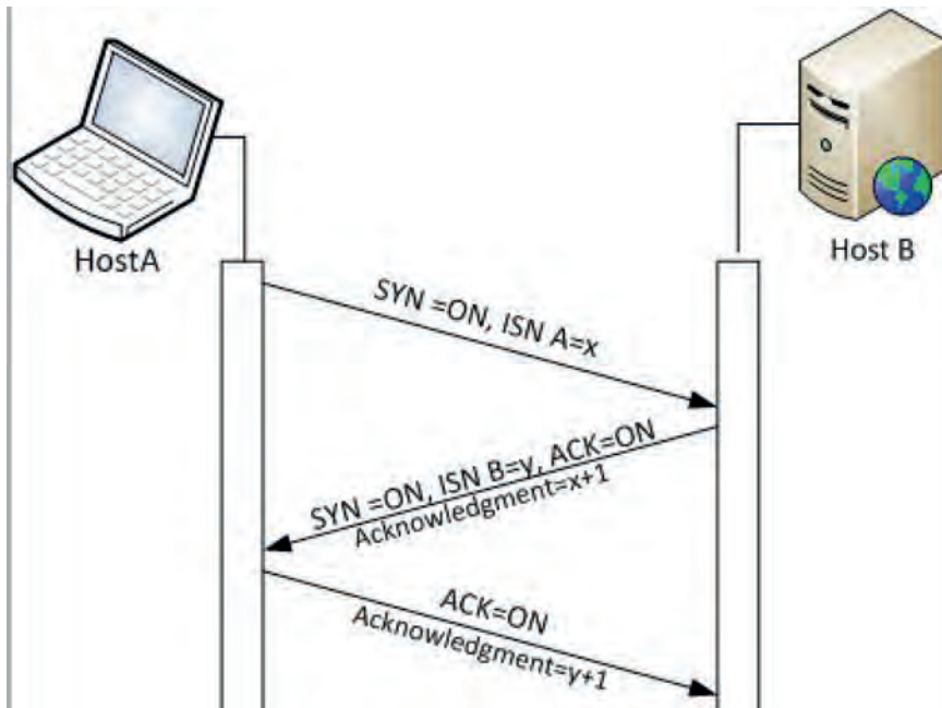
Εικόνα 4.3.α: Εγκατάσταση νέας Σύνδεσης με τριμερή χειραψία.
