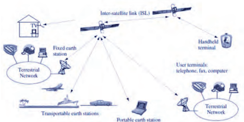
Σχήμα 5.3.2.α: Τυπικές εφαρμογές και υπηρεσίες δορυφορικής δικτύωσης (Πηγή: Zhili Sun, (2014), "Satellite networking principles and protocols")
