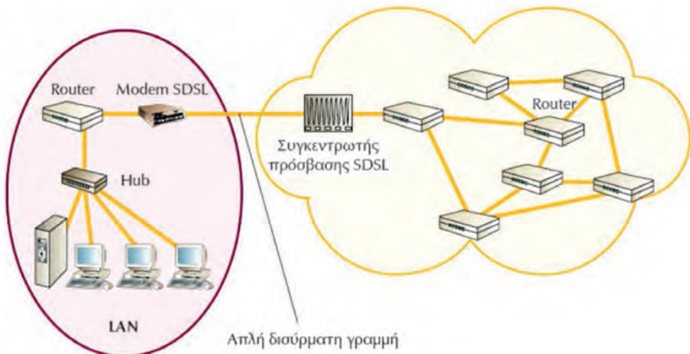
Σχήμα 5.1.4.α. Πρόσβαση τοπικού δικτύου σε δίκτυο ευρείας περιοχής με την τεχνολογία SDSL (Πηγή: Αρβανίτης, Κ., Κολυβάς, Γ., & Ούτσιος, Σ. (2001). Τεχνολογία Δικτύων Επικοινωνιών)
