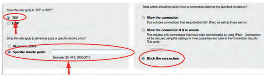
Εικόνα 7: Ορισμός φίλτρου
