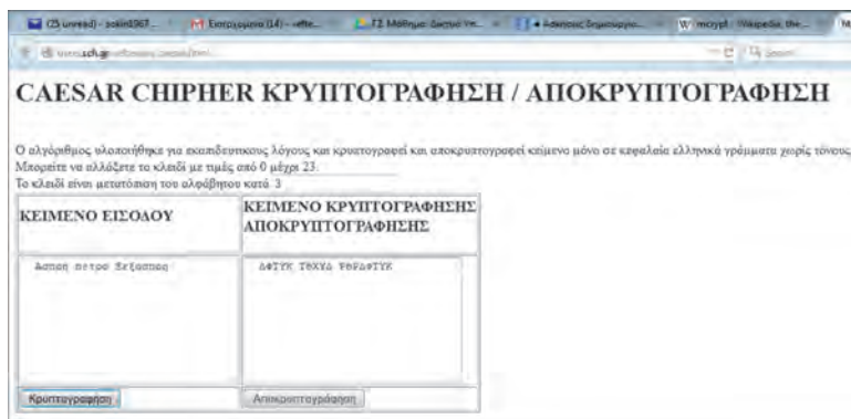
Εικόνα 10: Caesar Chipher
