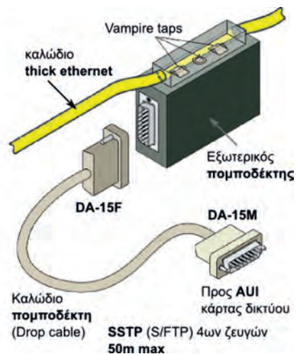
Εικόνα 2.4.1.β: Εξ. πομποδέκτης Thick Ethernet.
