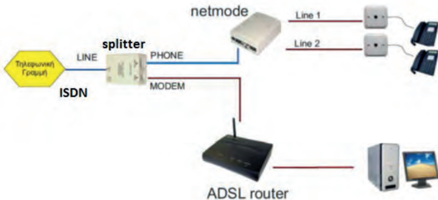
Σχήμα 5.1.4.2.δ. Σύνδεση ADSL σε γραμμή ISDN με χρήση διαχωριστή σήματος (splitter-based)
