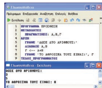
Εικόνα 1.4. Ο κώδικας για την άθροιση δύο αριθμών στο προγραμματιστικό περιβάλλον Γλωσσολάβεια
