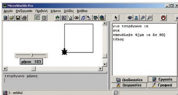
Εικόνα 2.7. Η διαδικασία τετράγωνο παίρνει τιμές από το μεταβολέα «μήκος».
